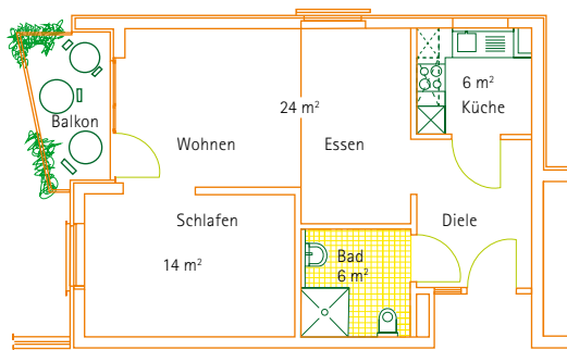
Grundriss Bugenhagenstraße (Gesamtfläche 50 m 2 ) Beispiel Wohnungstyp 3A
